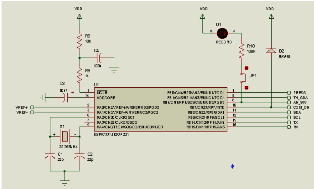
dsPIC33 Circuit section
